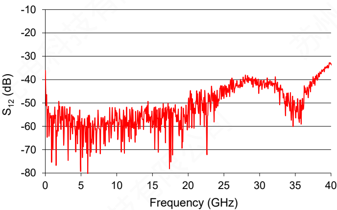
S_{12} Parameter Curve Conditions: V_{bias} = 8\text{ V} , V_{amp} = 1.5\text{ V} , V_{xp} = 2\text{ V} , I_{bias} = 300\text{ mA}
