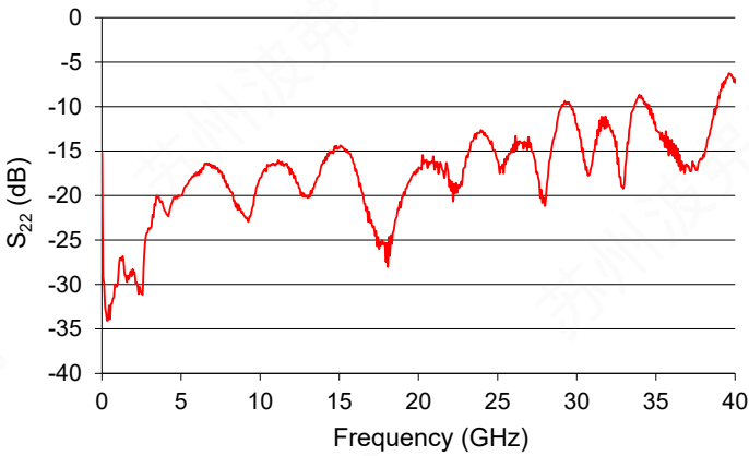
S_{22} Parameter Curve Conditions: V_{bias} = 8\text{ V} , V_{amp} = 1.5\text{ V} , V_{xp} = 2\text{ V} , I_{bias} = 300\text{ mA}
